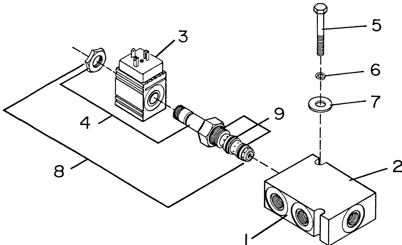
ASSEMBLY ITEMS 2,3,4
